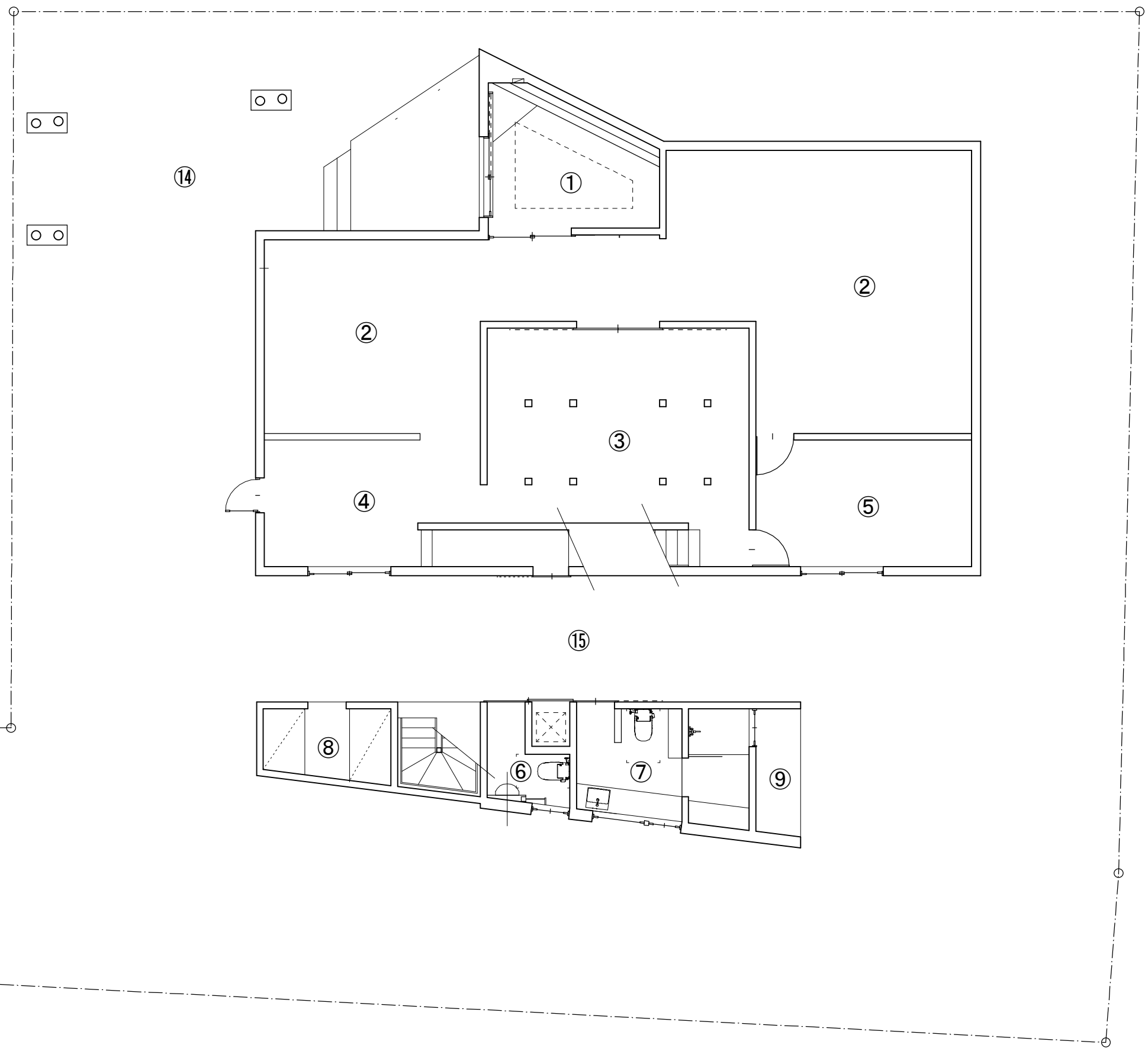
1階平面図
