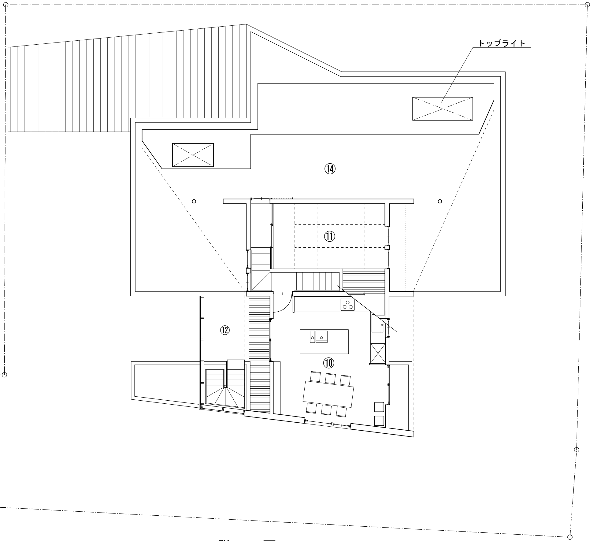
2階平面図
